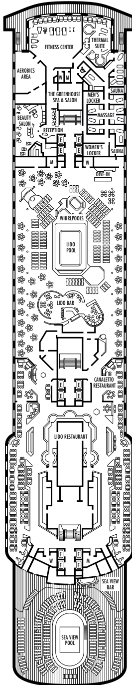
Lido-Deck
